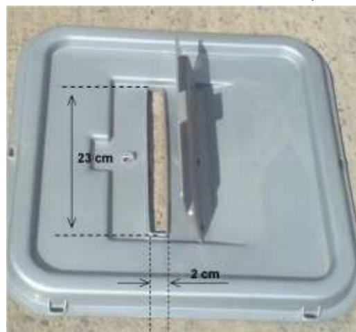
Figura nr. 7 Capacul cu fantă al urnei de vot staționară
