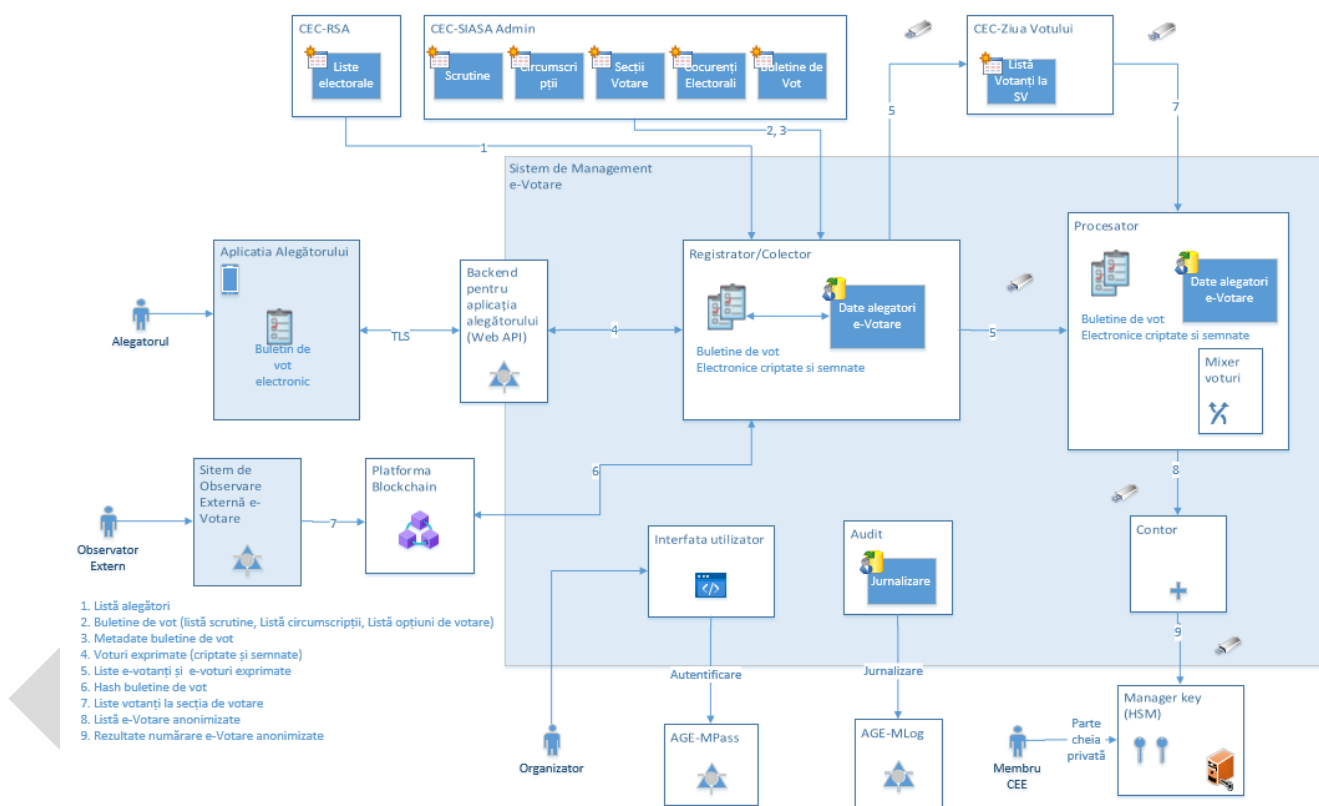
Figura 3. Sistemul de Management e-Votare și interacțiunea cu alte aplicații, steme și servicii.
