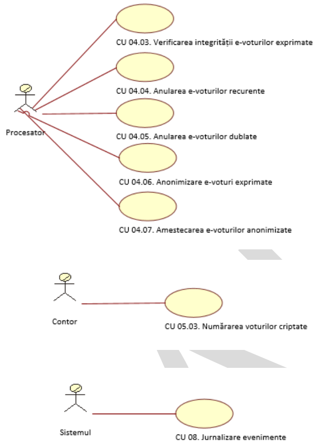
Figura 9. Diagramele cazurilor de utilizare aferent Actorilor nonumani.
